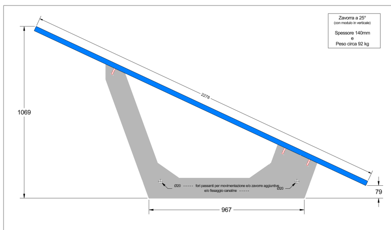
Quote con modulo di lato 2278mm
