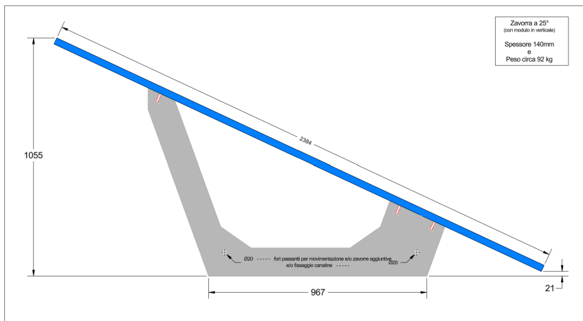
Quote con modulo di lato 2384mm
