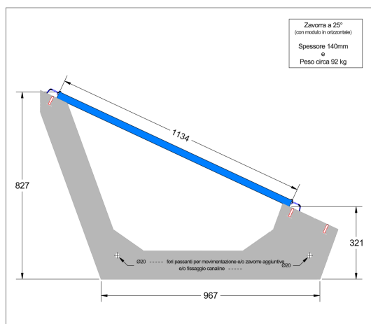
Quote con modulo di lato 1134mm
